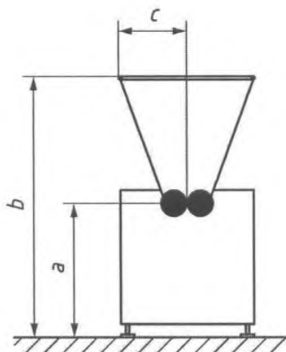
Рисунок 13 — Загрузочный бункер с предохранительными планками с реакцией на давление
