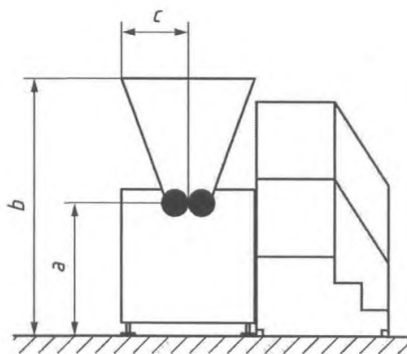
Рисунок 9 — Заблокированные ступеньки и рабочая площадка
