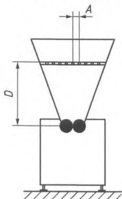
Рисунок 7 — Неподвижное защитное ограждение
