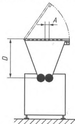
Рисунок 6 — Защитное ограждение с отверстиями (решетка) с блокирующим устройством
