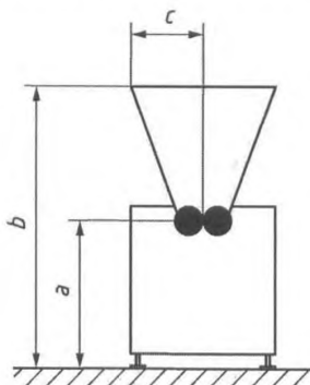
Рисунок 8 — Защита безопасным расстоянием
