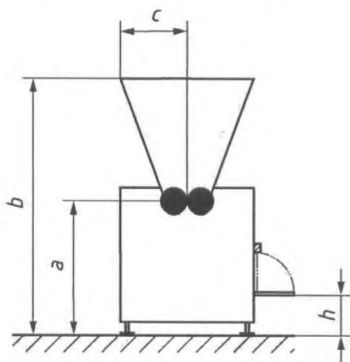
Рисунок 10 — Бункер с заблокированным откидным трапом
