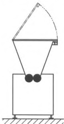
Рисунок 5 — Жесткое защитное ограждение с блокирующим устройством
