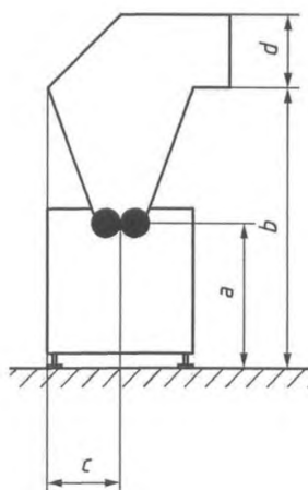
Рисунок 11 — Питающий бункер с воротниковой воронкой
