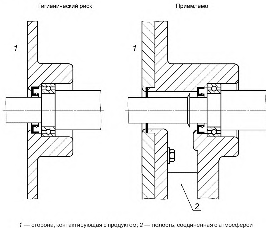
Рисунок В.9 — Конструкция входа вала
