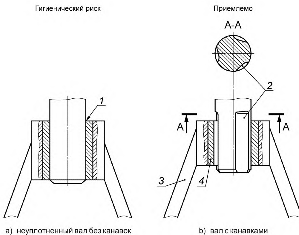
Рисунок В.10 — Подшипники, смазываемые продуктом
