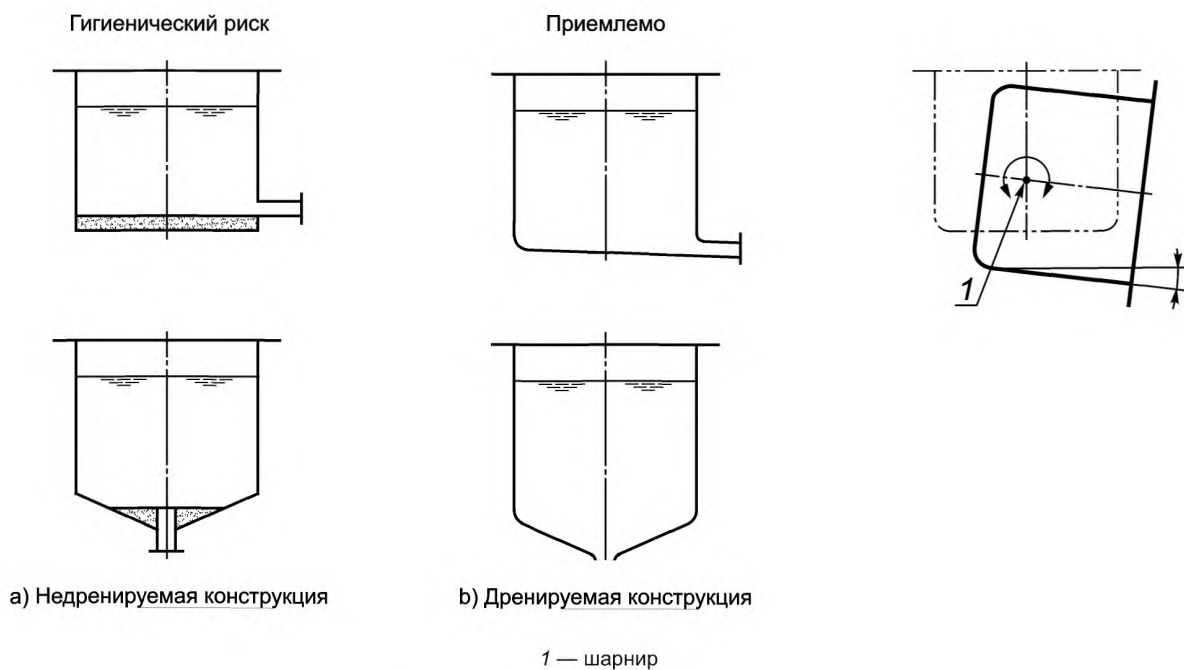
Рисунок В.1 — Дренирование сосудов
