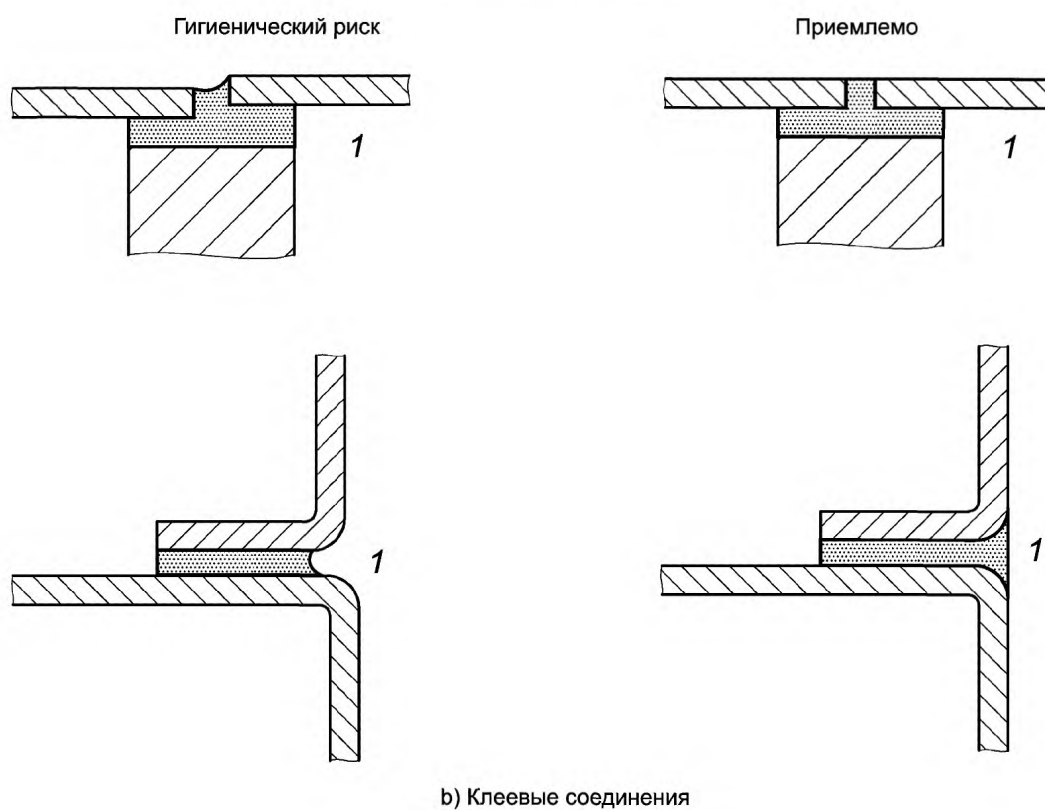
Рисунок В.4 — Постоянные соединения
