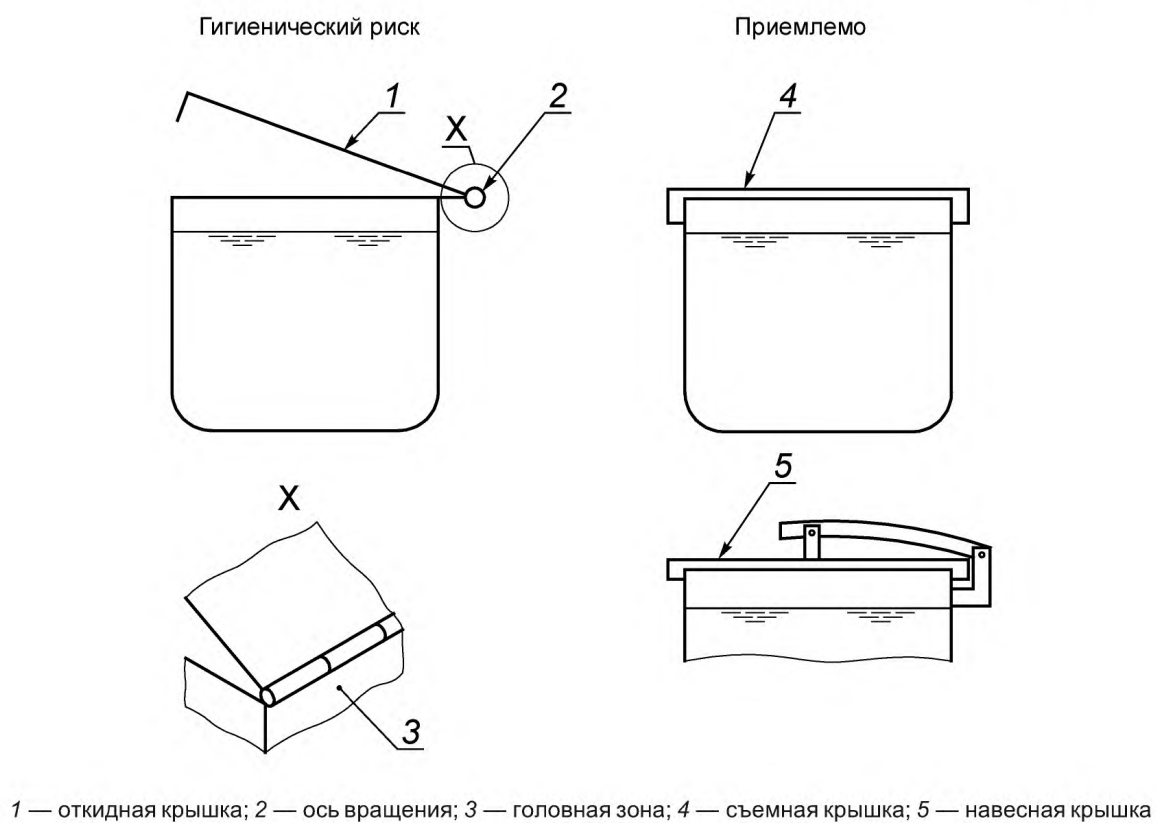
Рисунок В.11 — Проемы и крышки
